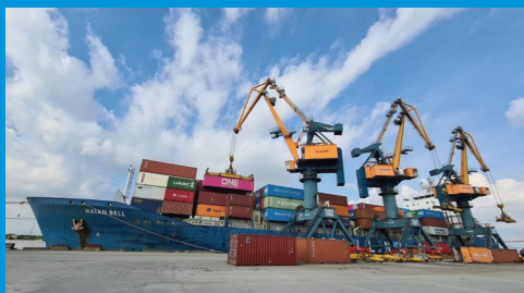
Trang bị 03 cần cẩu 45 tấn với tổng năng suất xếp dỡ 75 move/giờ, 14 xe nâng và các thiết bị khác phục vụ khai thác tàu và kho bãi. Equipped with three 45-ton cranes with a total throughput of 75 moves/hour, 14 reach stackers, and other equipment for vessel and CY operation.
